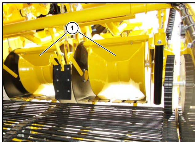
(1) Abstreifer Dammrolle
