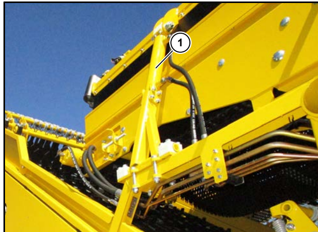
(1) Zylinder Igelband 4 Neigung
