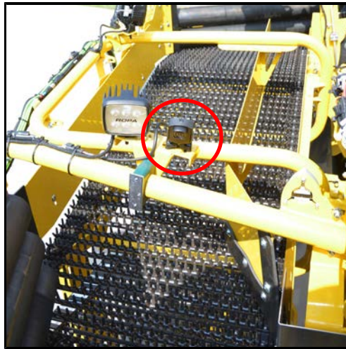
Digitalkamera Igel 1 und 2
