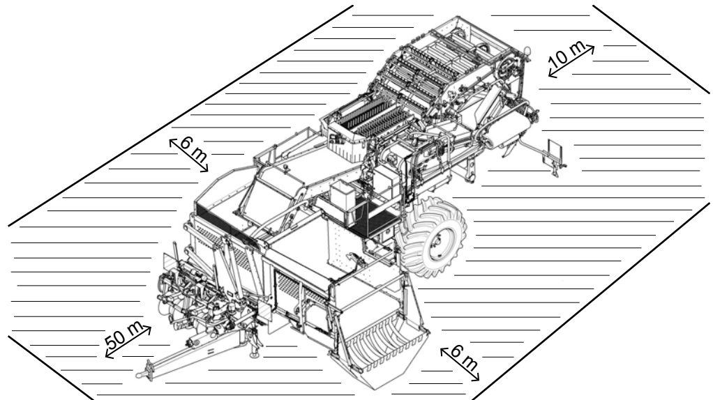
Gefahrenbereich Bunkermaschine
