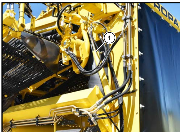
(1) Zylinder Igelband 1/2 Neigung
