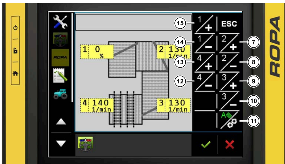
Igelautomatik aktiviert
