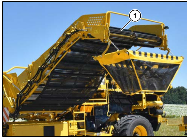
(1) Entladeband Überladerbunker
