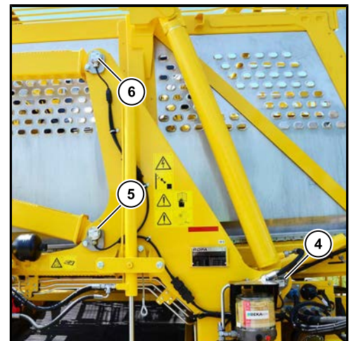
Ansicht Bunker von vorne
