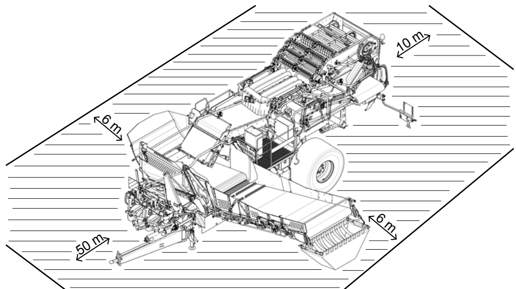
Beispiel Gefahrenbereich Überladerbunkermaschine
