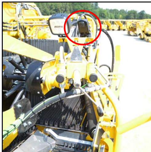
Digitalkamera Beimengenband DoubleSelect
