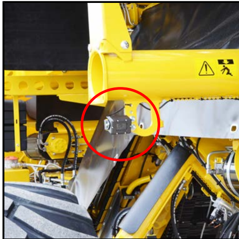
Videokamera Schmutzaustrageband
