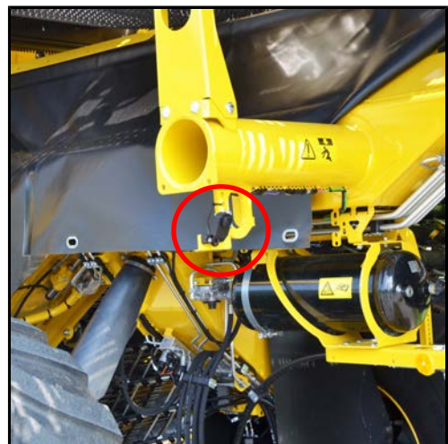
Digitalkamera Schmutzaustrageband
