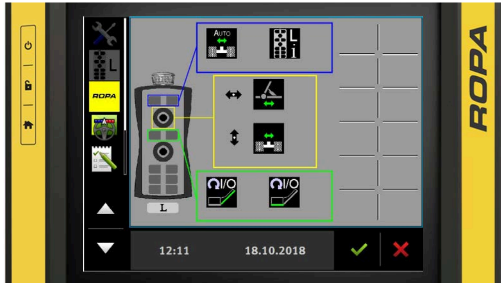
Anzeige oben
