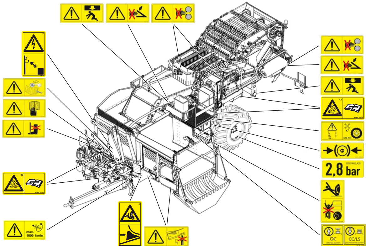
Bunkermaschine Ansicht links vorne
