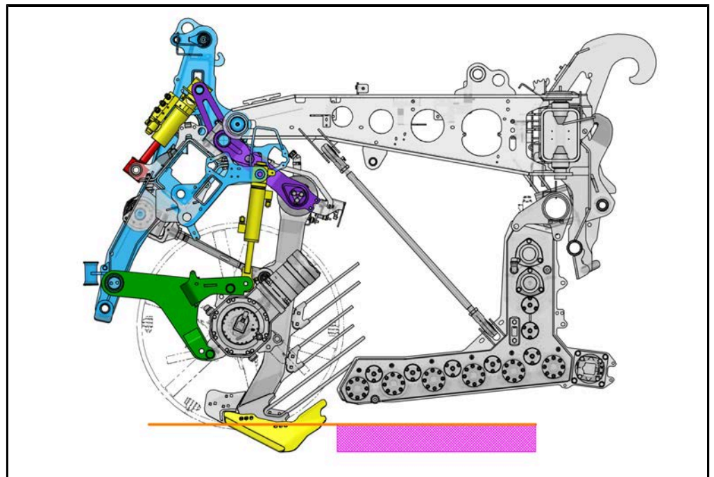
Schartiefe tief
