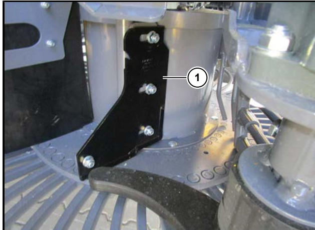
(1) Siebsterne Abstreifer
