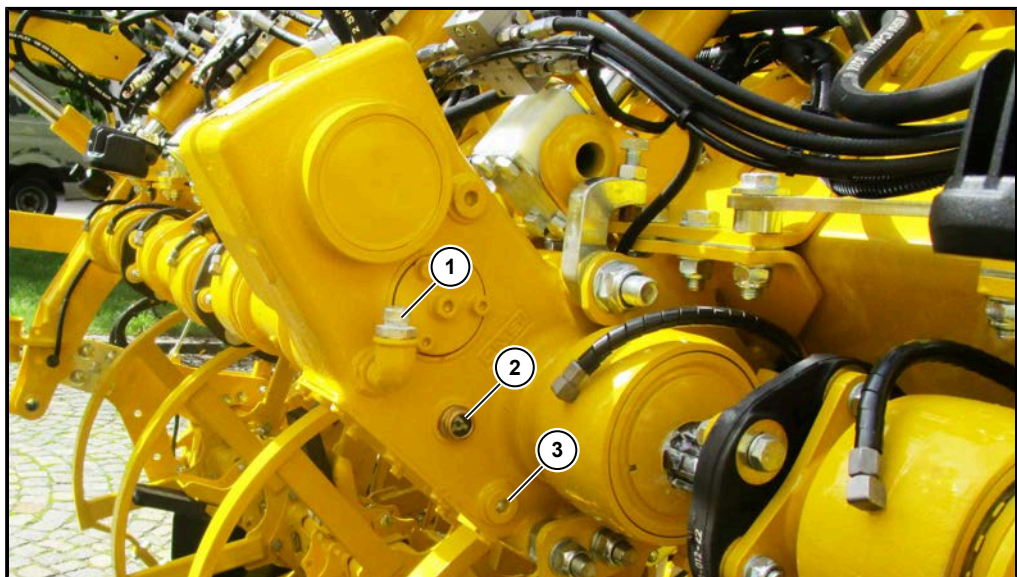
Bild zeigt Ausführung ab 2017
