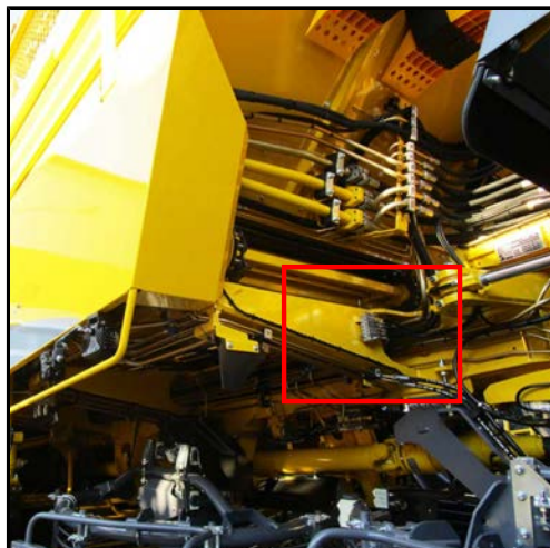
Hauptverteiler Fahrgestell
