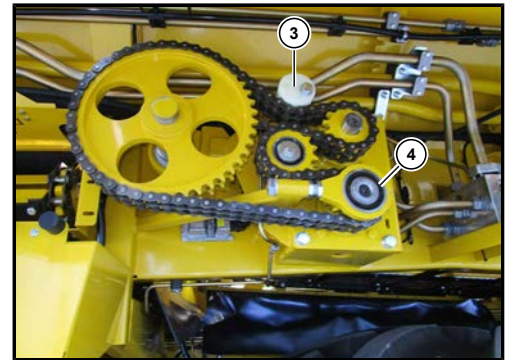
Antriebskette Längskratzboden
