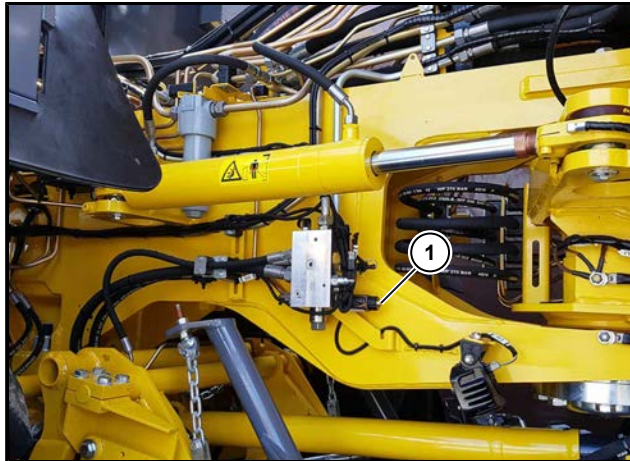
(1) Steuerblock Siebband
