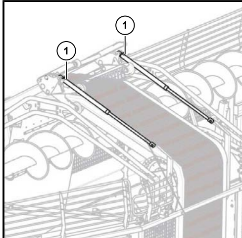
(1) Stützzylinder
