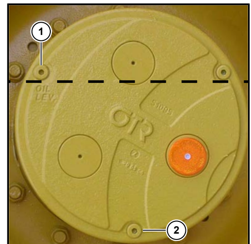
Planetengetriebe Hinterachsen
