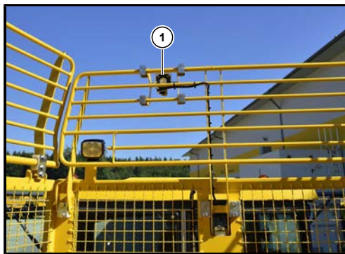
(1) Ultraschallsensor vorne
