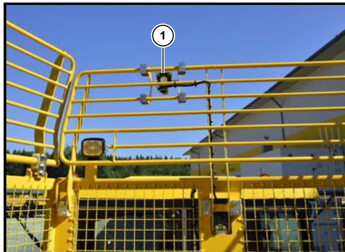
(1) Ultraschallsensor vorne
