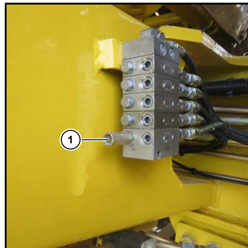
(1) Hubstift
