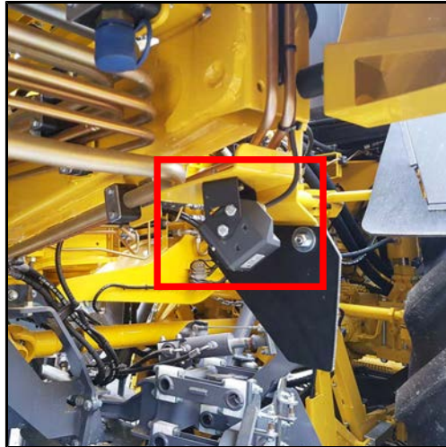
Siebsternkamera
