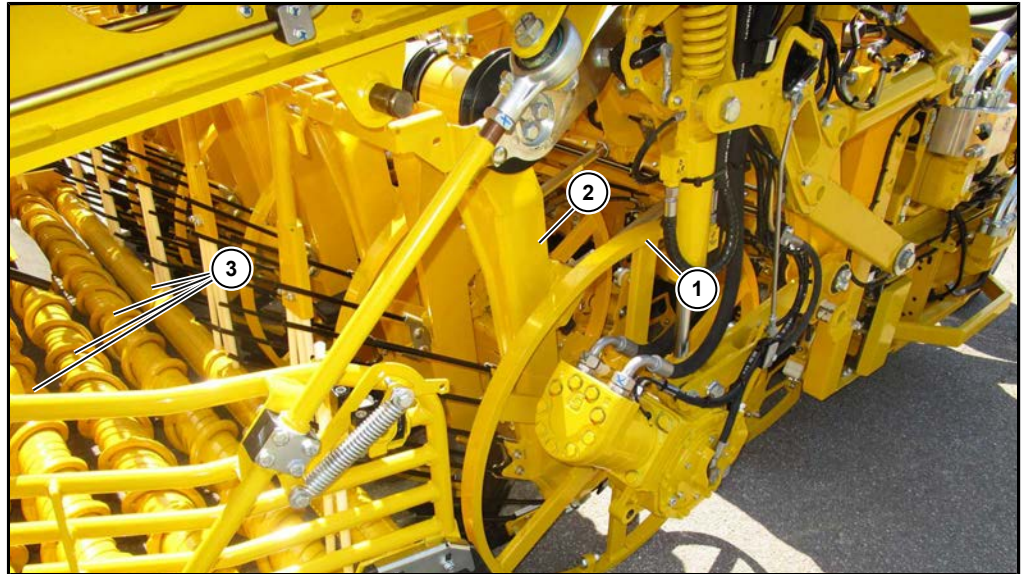
Rodeaggregate, zur besseren Übersicht ohne Schutzvorrichtung abgebildet
