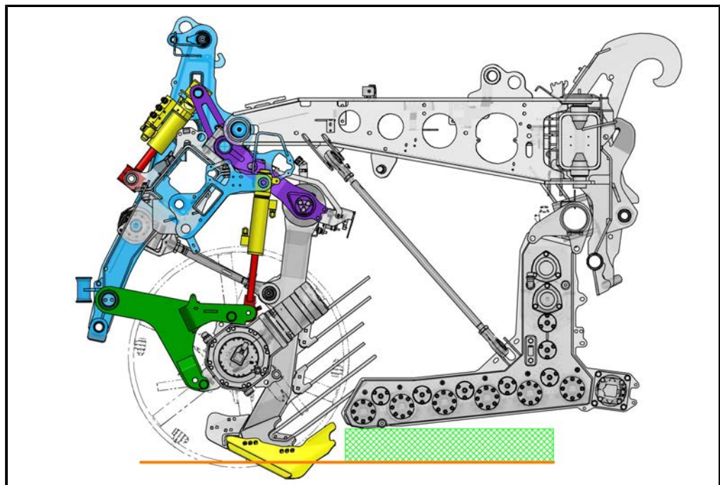
Walzengang hoch
