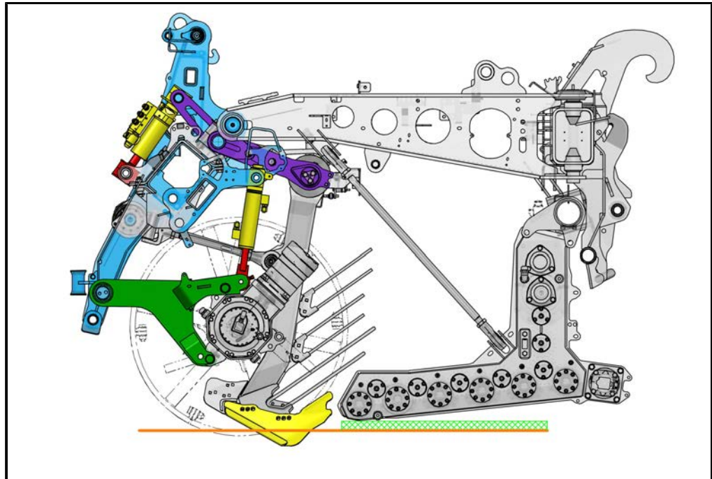
Walzengang tief
